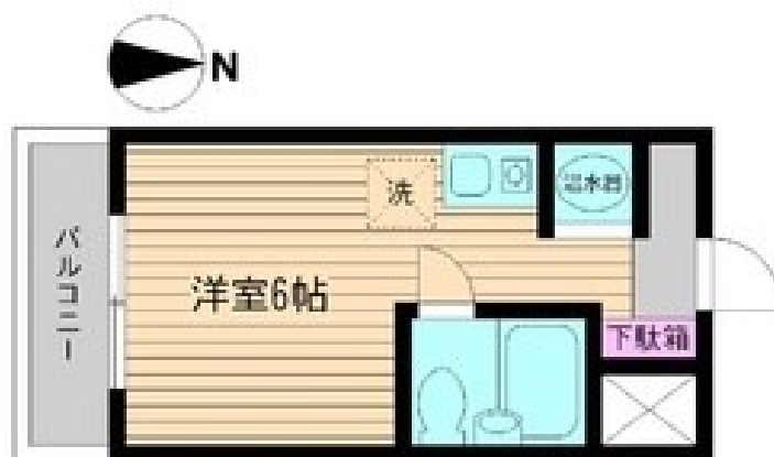
【間取り図】
