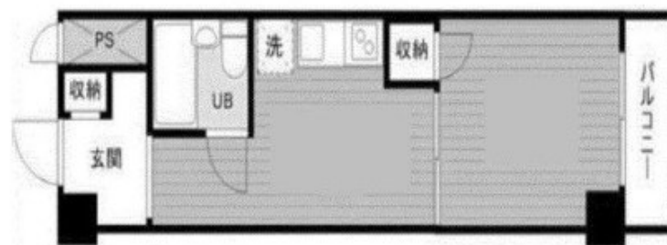
【間取り図】
