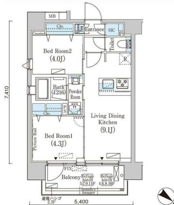
【間取り図】
