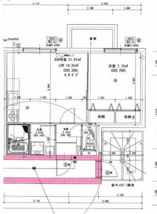
【間取り図】
